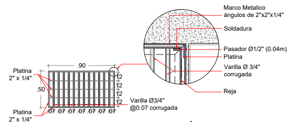
DETALLE REJA METÁLICA
