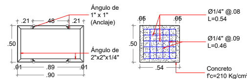
DETALLE MARCO PARA REJA 0.50 x 0.90
