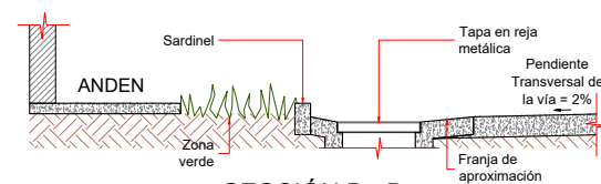
SECCIÓN B - B
